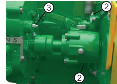
Cojinetes de los ejes de accionamiento (2) y del engranaje de la caja selectora (3)
